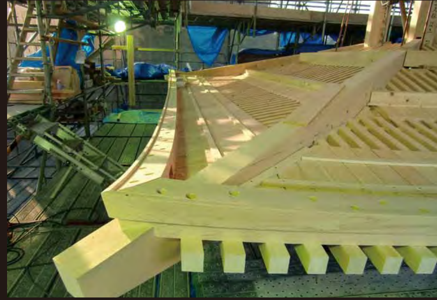
19 茅負反り
