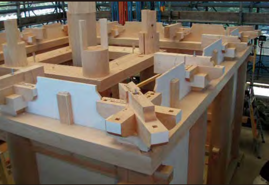
08 肘木取付
