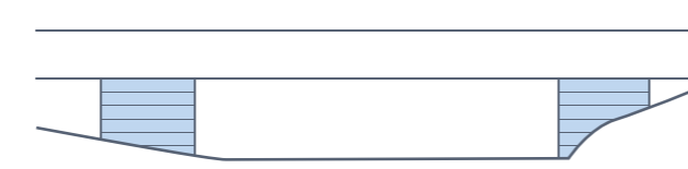
1. 橋脚を鉄板で巻いて補強する
