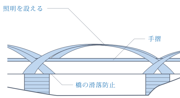
2. 糸に見立てた鉄板を橋脚から伸ばす
