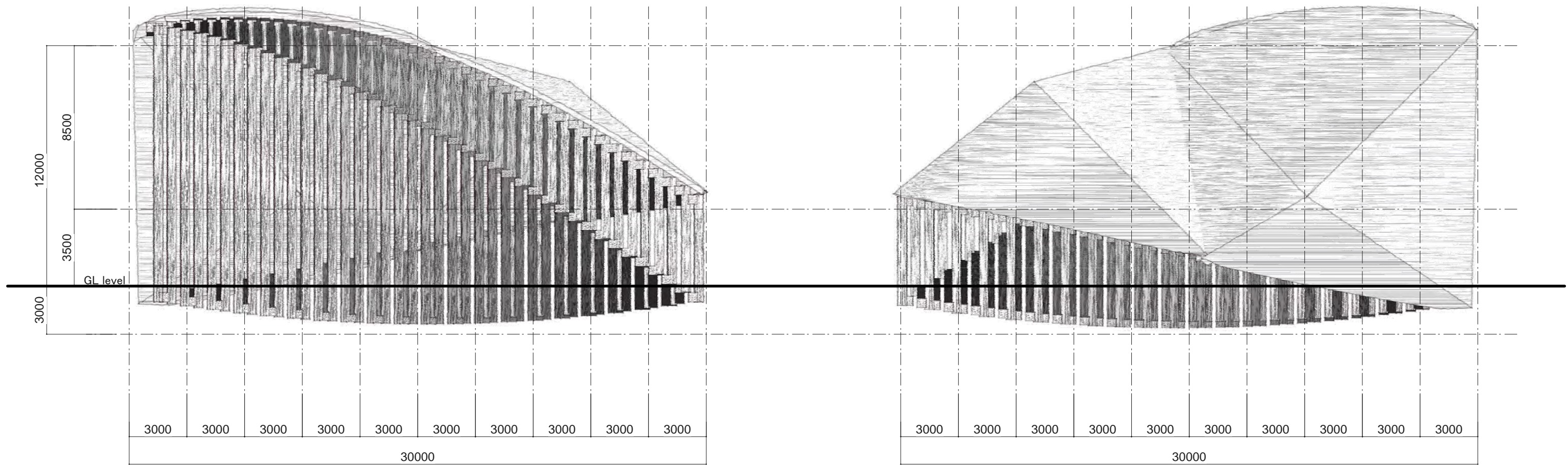
西立面图
