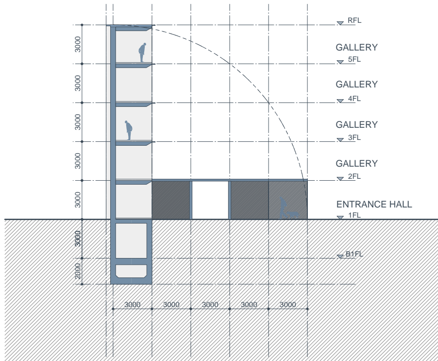
SECTION A-A 1/200
